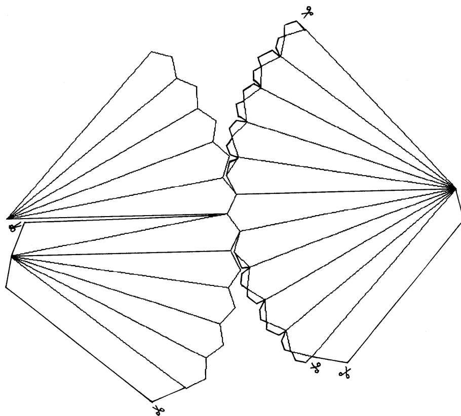
Solide de Johnson – Antidiamant décagonal
